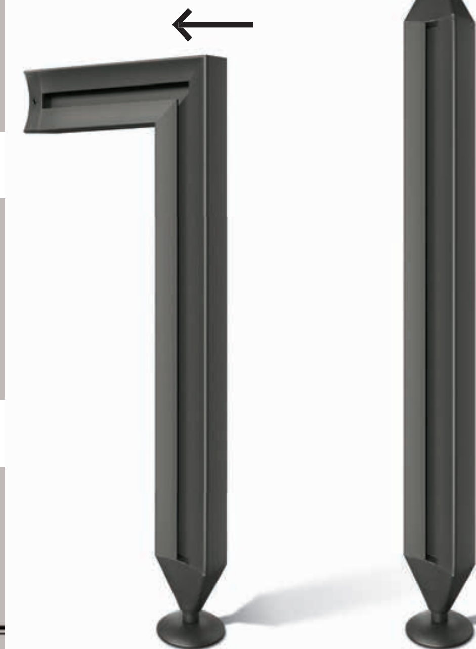
articolo 4051 montante in metallo con piedino parte finale per fissaggio a muro. metal upright with final foot for wall fixing. cm. h. 260
